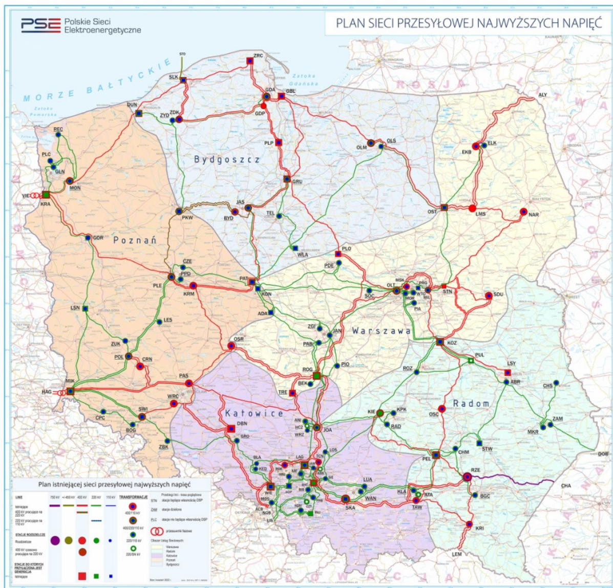
Okręgi sieci przesyłowej najwyższych napięć. Źródło: Polskie Sieci Elektroenergetyczne S.A.
